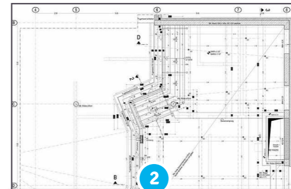
2 Grundriss & Bemaßung durch den Schwimmbadbauer/Architekten
